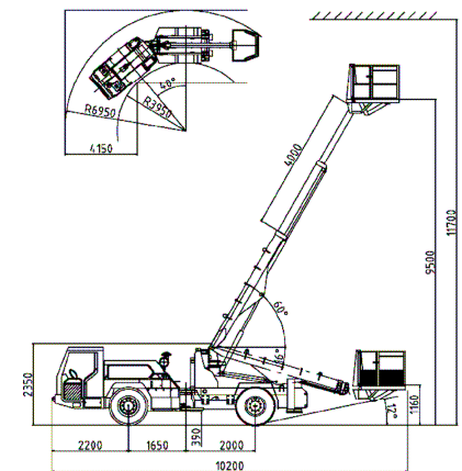
als Hubbühne – 500 kg
