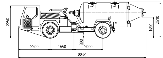
als Betonmischer – 5 m 3
